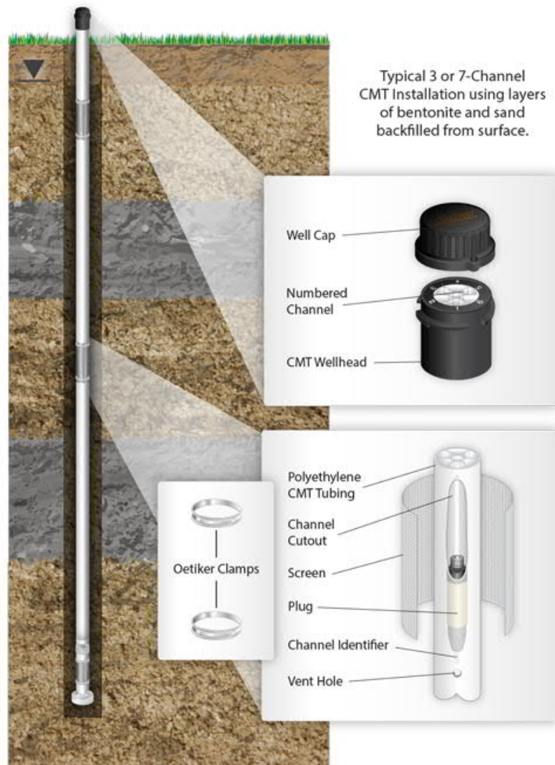
Figure 19 : Système CMT (source : https://www.solinst.com/ )
