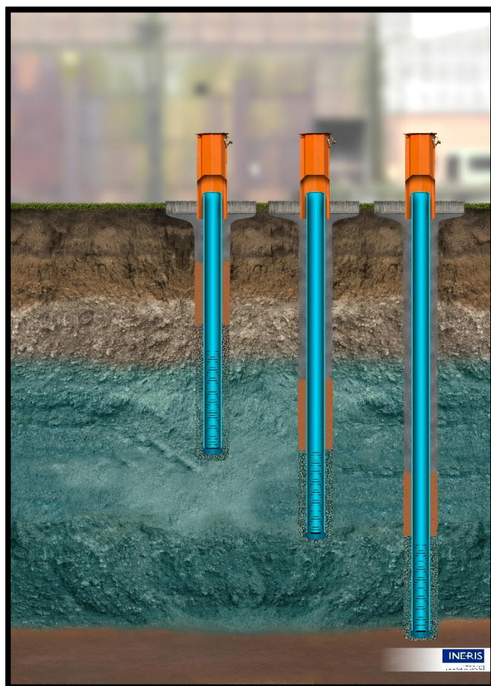
Figure 8 : Plusieurs piézomètres à différentes profondeurs (flûte de pan ou « Cluster Well »)
