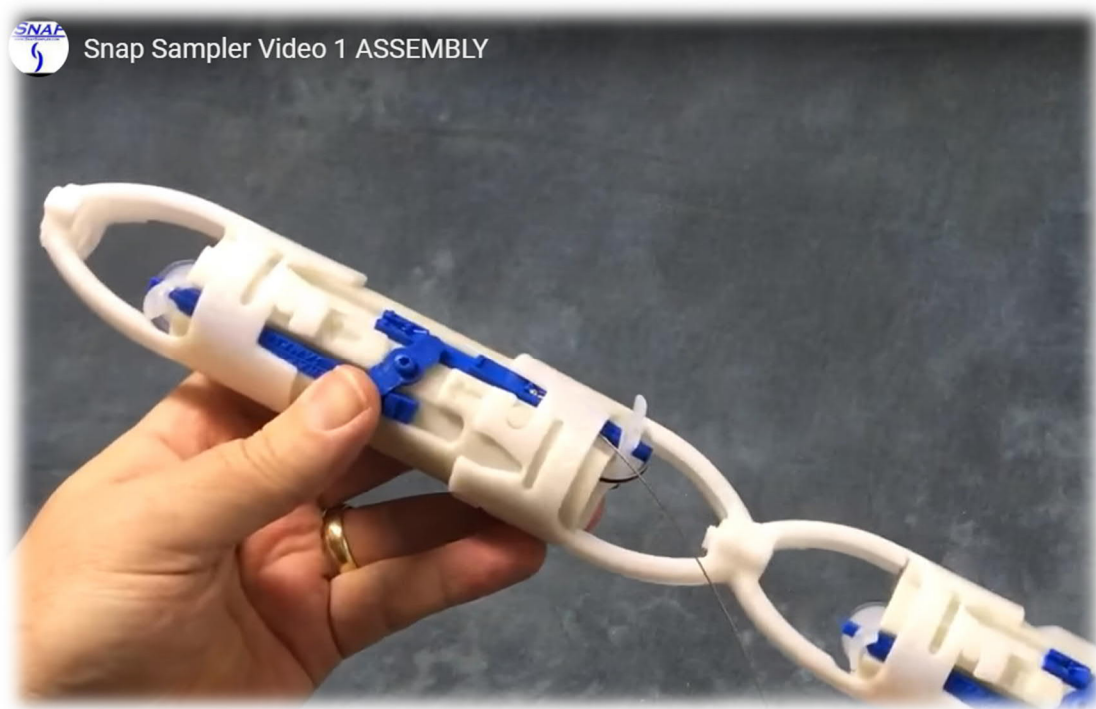
Figure 18 : Echantillonneur Snap Sampler composé de plusieurs bouteilles de prélèvements (source : http://snapsampler.com/ )
