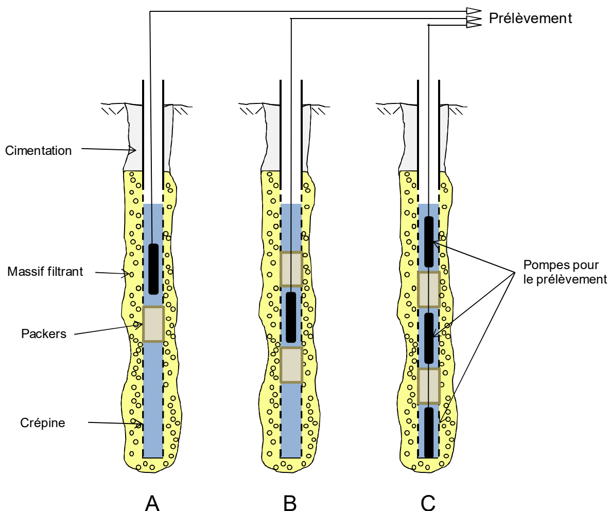
Figure 14 : Différentes configurations pour l'utilisation des packers (avec pompes immergées par exemple) ; A- Prélèvement au toit de la nappe (1 pompe) ; B – Prélèvement entre packers (1 pompe) ; C- Prélèvement de 3 niveaux (3 pompes) (source : Ineris)
