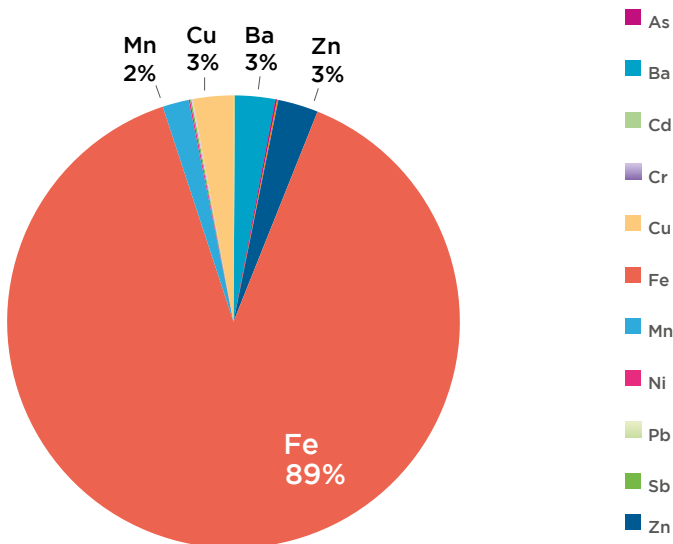
Figure 10: Répartition des métaux présents dans l'air en EFS sur quai
