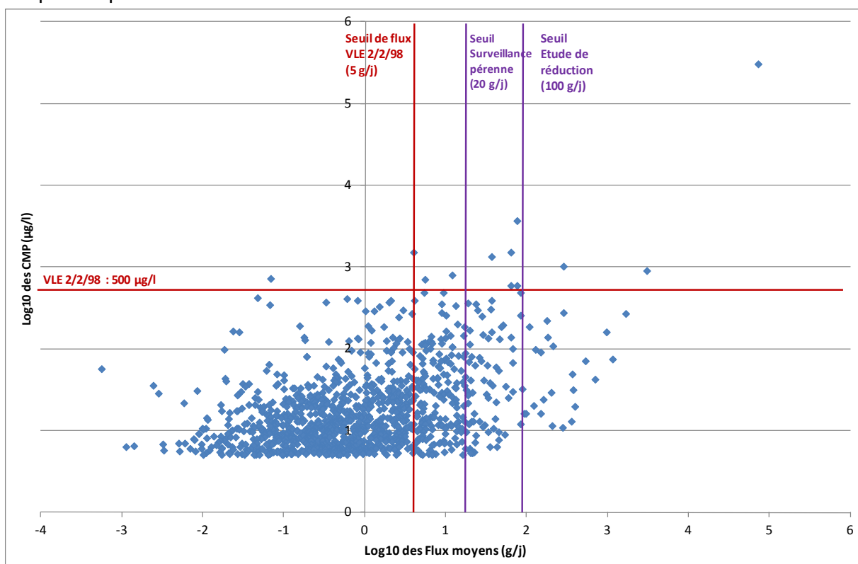
Figure 23 : Niveaux d'émission de plomb sur l'ensemble des points de rejet (concentrations moyennes pondérées en fonction des flux moyens)
