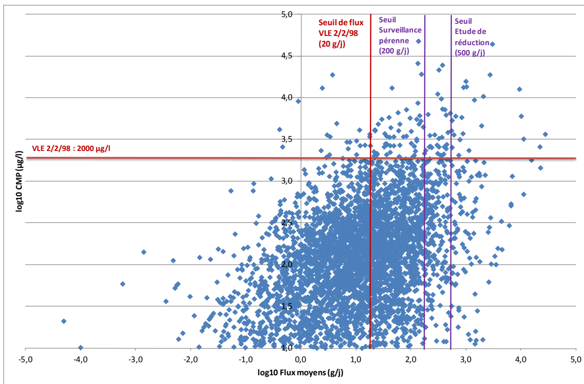
Figure 12 : Niveaux d'émission de zinc sur l'ensemble des points de rejet (concentrations moyennes pondérées en fonction des flux moyens)
