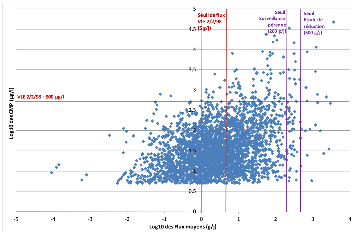
Figure 15 : Niveaux d'émission de cuivre sur l'ensemble des points de rejet (concentrations moyennes pondérées en fonction des flux moyens)
