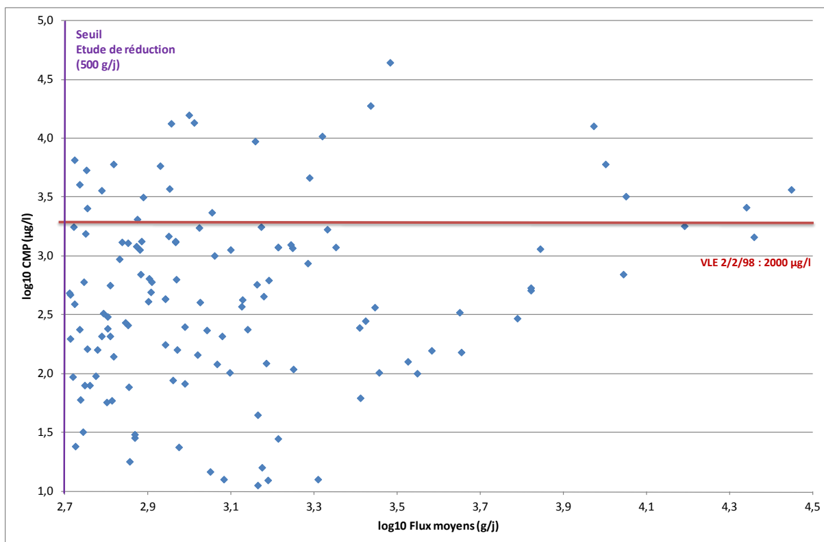
Figure 13 : Niveaux d'émission de zinc sur les points de rejet dépassant les seuils d'études de réduction (concentrations moyennes pondérées en fonction des flux moyens)
