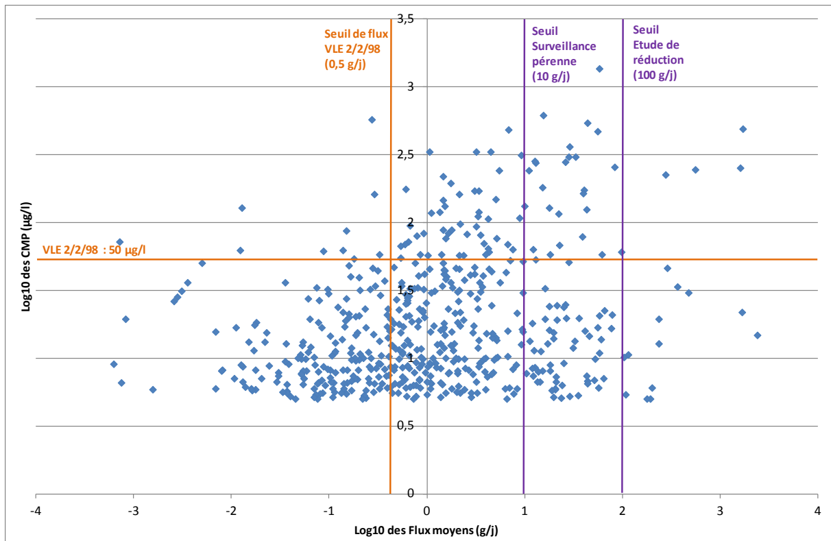
Figure 21 : Niveaux d'émission d'arsenic sur l'ensemble des points de rejet (concentrations moyennes pondérées en fonction des flux moyens)
