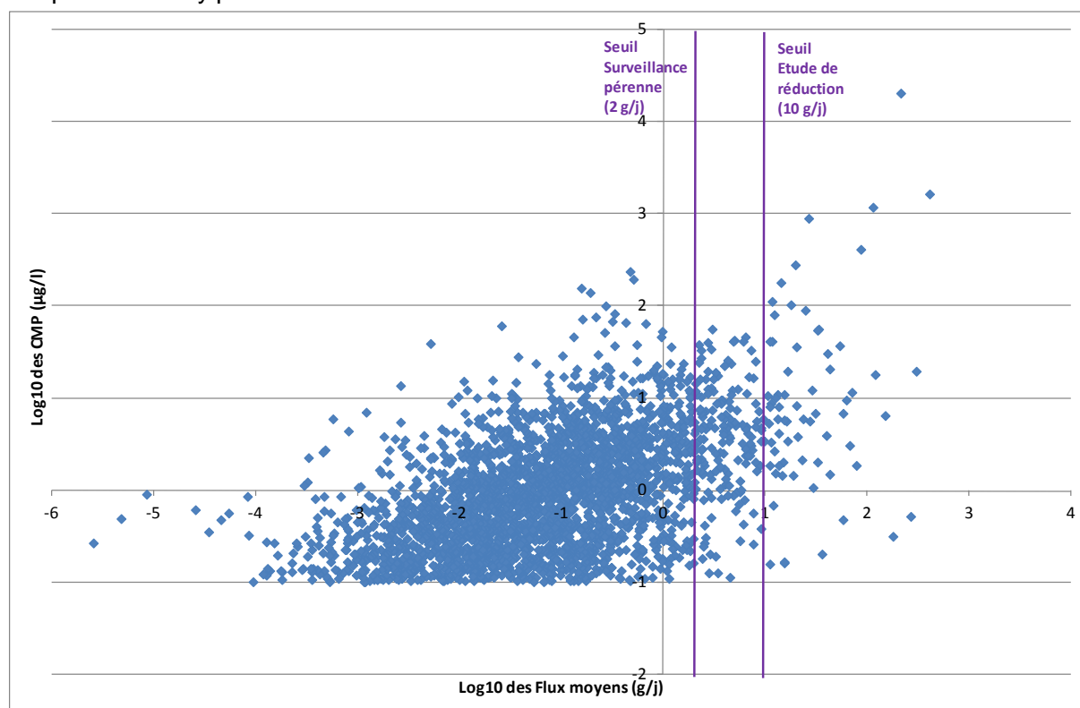
Figure 28 : Niveaux d'émission de nonylphénols sur l'ensemble des points de rejet (concentrations moyennes pondérées en fonction des flux moyens)
