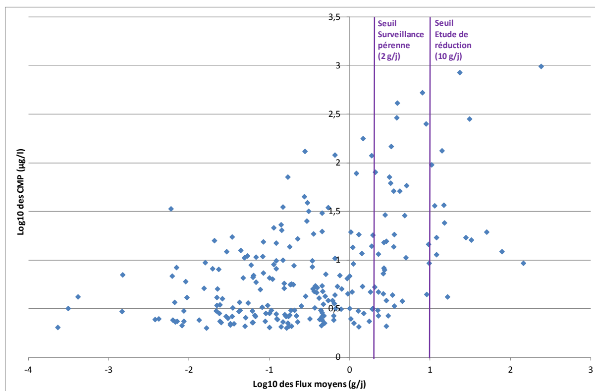
Figure 25 : Niveaux d'émission de cadmium sur l'ensemble des points de rejet (concentrations moyennes pondérées en fonction des flux moyens)
