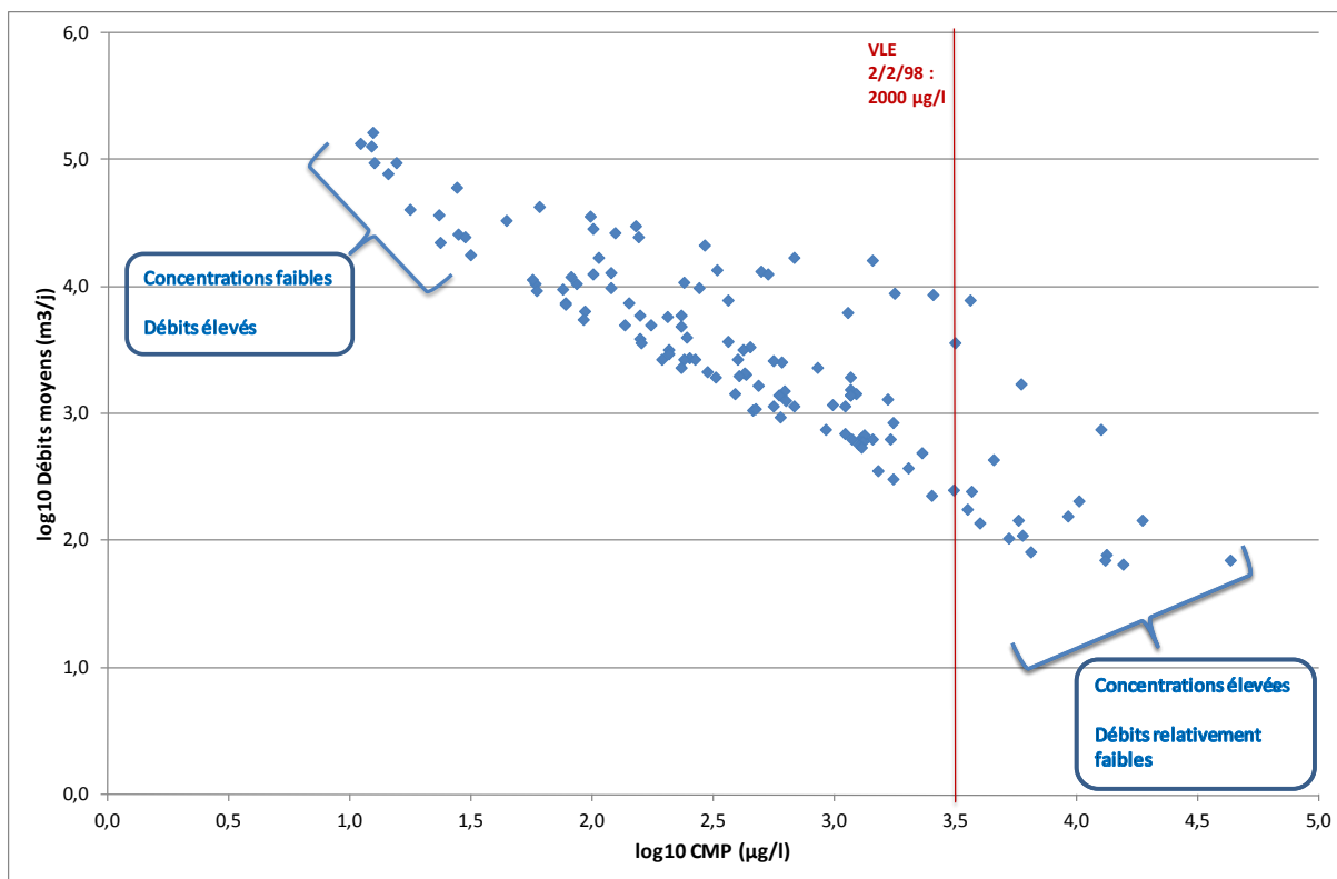
Figure 14 : Niveaux d'émission de zinc sur les points de rejet dépassant les seuils d'études de réduction (débits moyens en fonction des concentrations moyennes pondérées)
