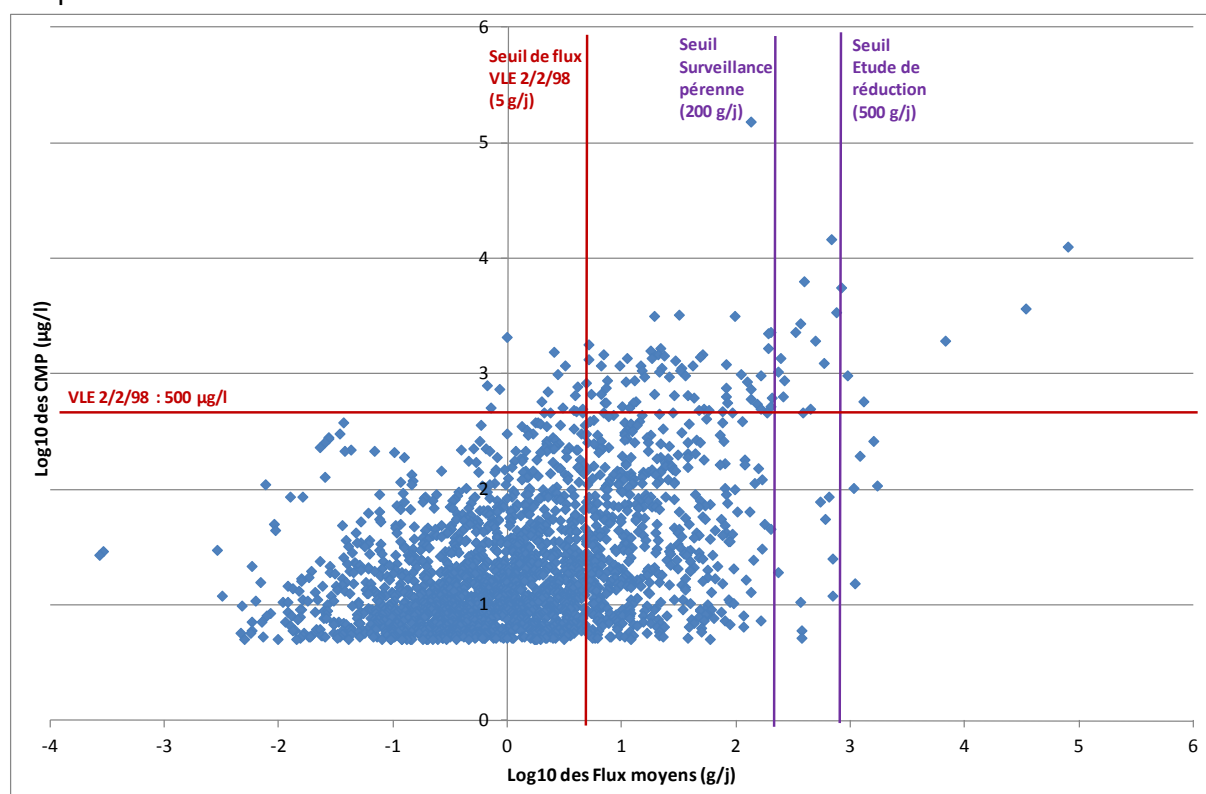
Figure 19 : Niveaux d'émission de chrome sur l'ensemble des points de rejet (concentrations moyennes pondérées en fonction des flux moyens)
