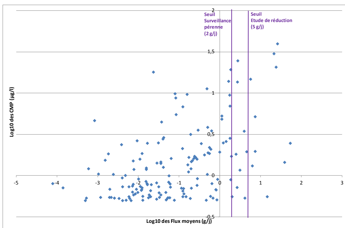
Figure 26 : Niveaux d'émission de mercure sur l'ensemble des points de rejet (concentrations moyennes pondérées en fonction des flux moyens)
