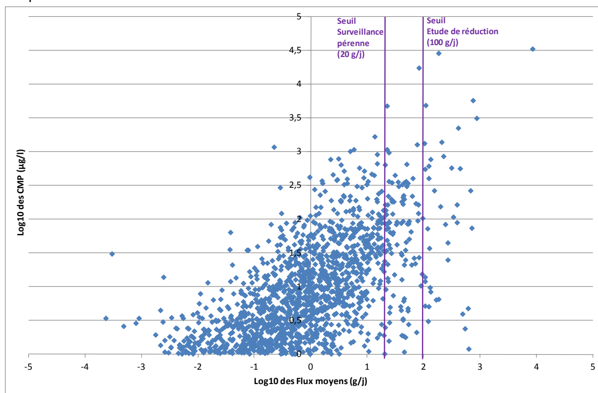
Figure 27 : Niveaux d'émission de chloroforme sur l'ensemble des points de rejet (concentrations moyennes pondérées en fonction des flux moyens)
