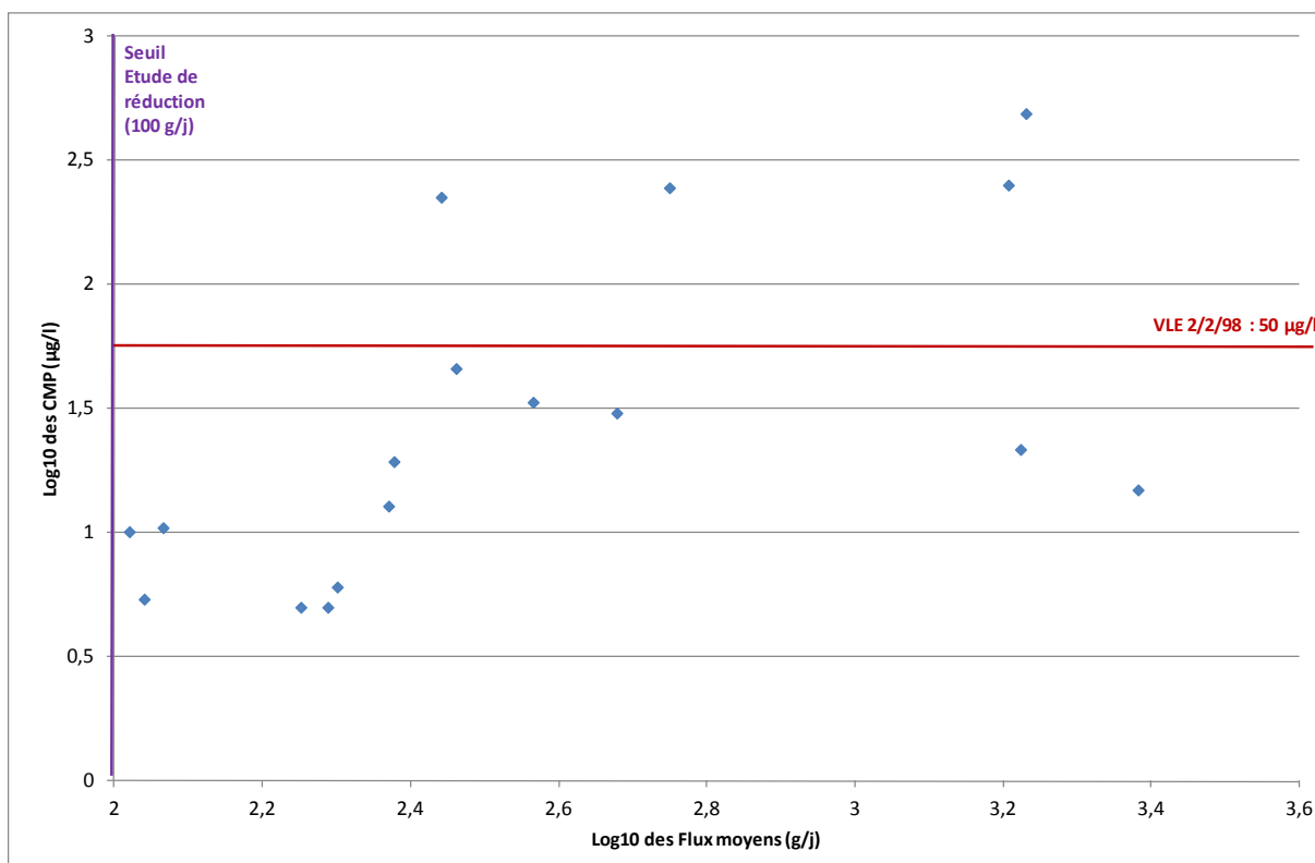
Figure 22 : Niveaux d'émission d'arsenic sur les points de rejet dépassant les seuils d'études de réduction (concentrations moyennes pondérées en fonction des flux moyens)
