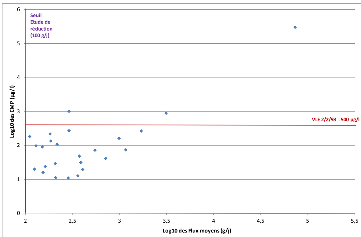
Figure 24 : Niveaux d'émission de plomb sur les points de rejet dépassant les seuils d'études de réduction (concentrations moyennes pondérées en fonction des flux moyens)
