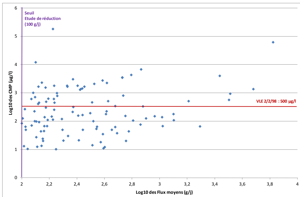
Figure 18 : Niveaux d'émission de nickel sur les points de rejet dépassant les seuils d'études de réduction (concentrations moyennes pondérées en fonction des flux moyens)
