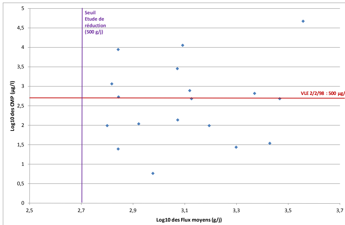
Figure 16 : Niveaux d'émission de cuivre sur les points de rejet dépassant les seuils d'études de réduction (concentrations moyennes pondérées en fonction des flux moyens)
