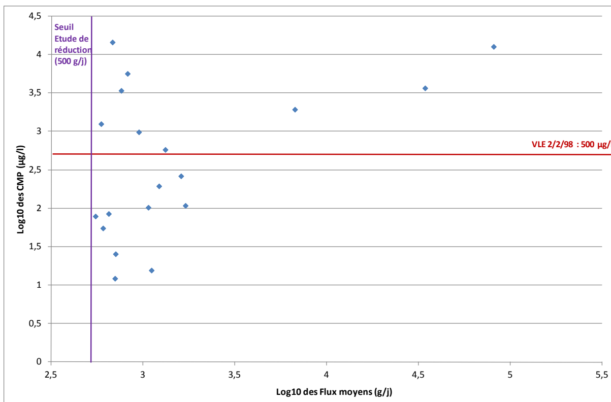
Figure 20 : Niveaux d'émission de chrome sur les points de rejet dépassant les seuils d'études de réduction (concentrations moyennes pondérées en fonction des flux moyens)
