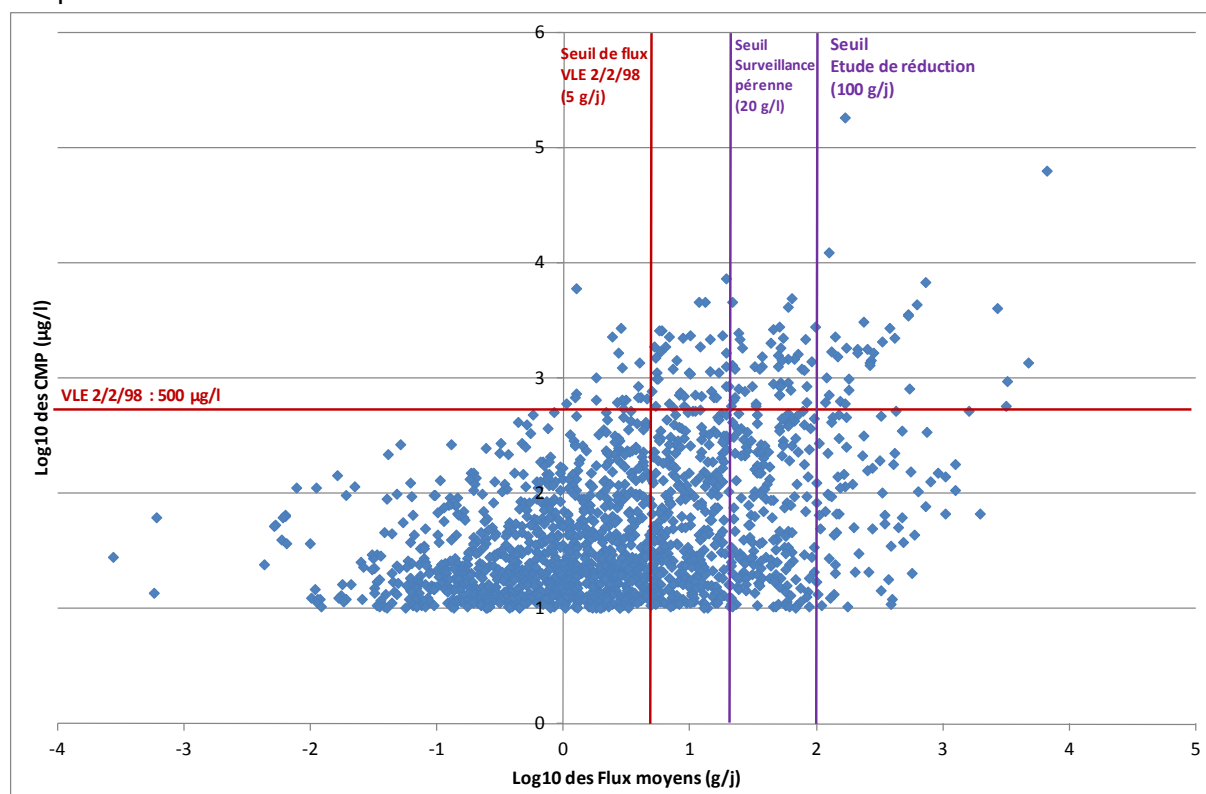
Figure 17 : Niveaux d'émission de nickel sur l'ensemble des points de rejet (concentrations moyennes pondérées en fonction des flux moyens)
