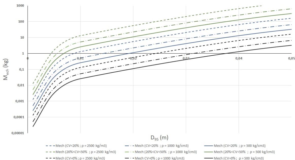
Figure 5 : Evolution de la masse d'un échantillon en fonction de sa granulométrie
