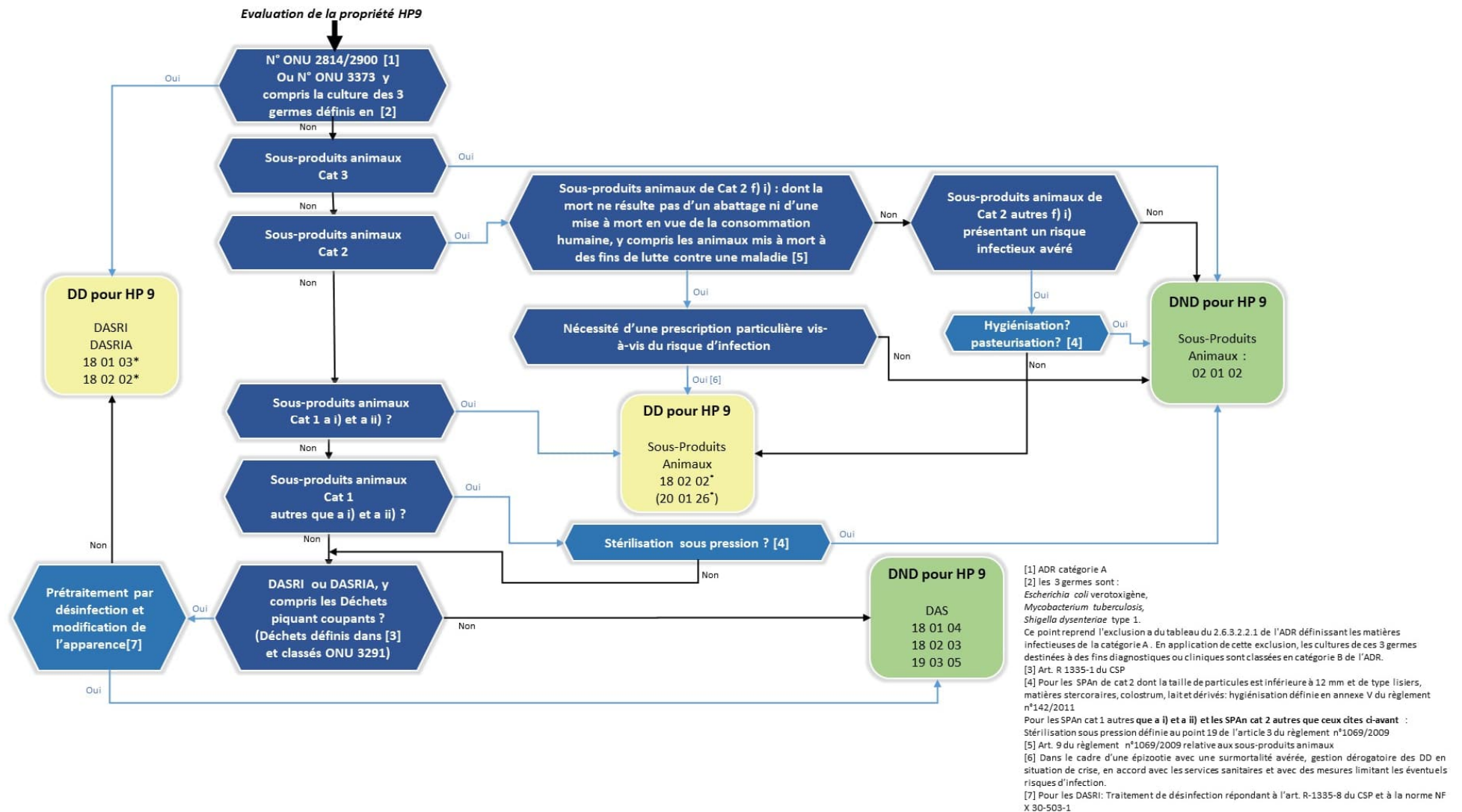
Figure 6 : Logigramme d'attribution de la propriété HP 9
