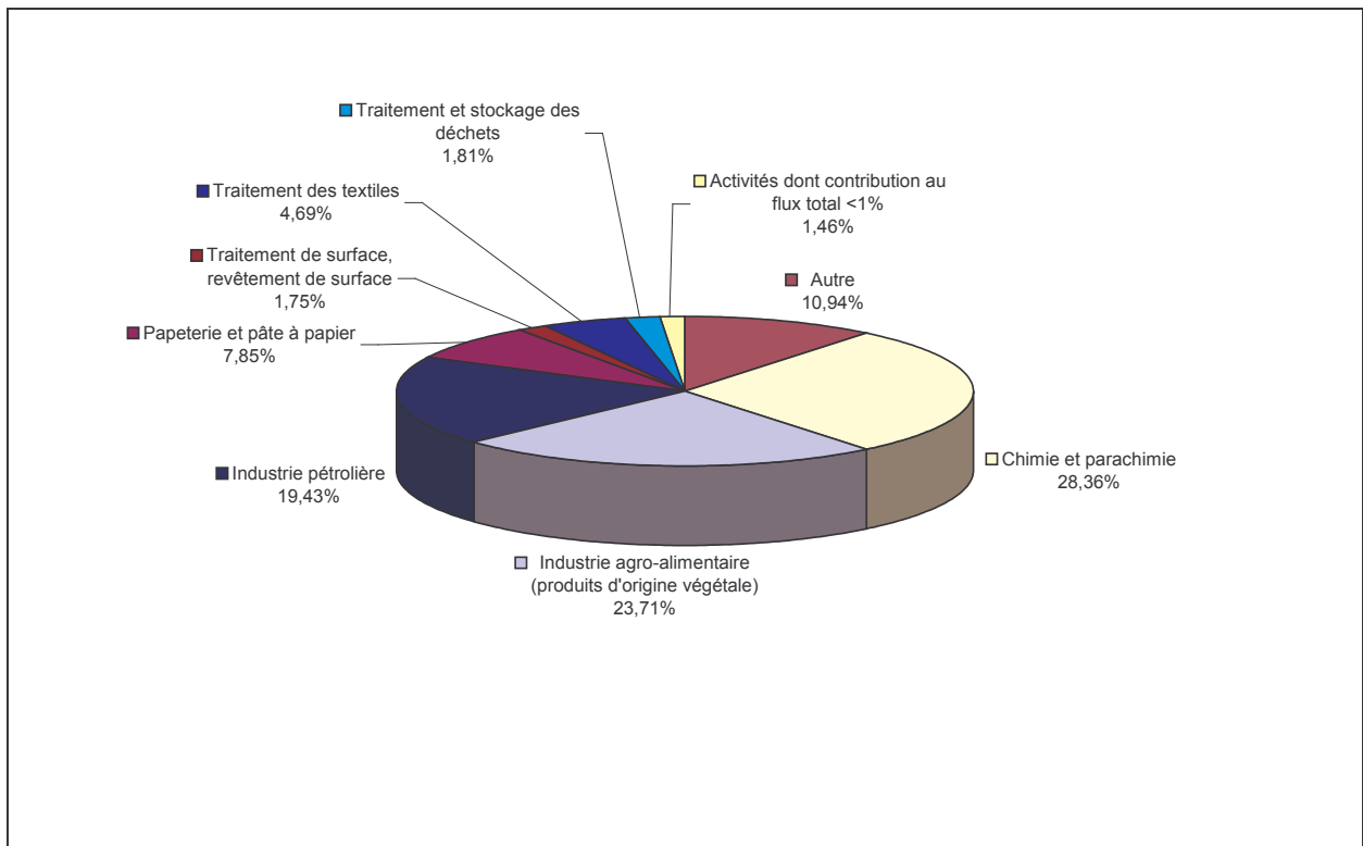
Figure 102 : Répartition par secteur d'activité des flux cumulés de PCB101 mesurés en sortie des sites industriels
