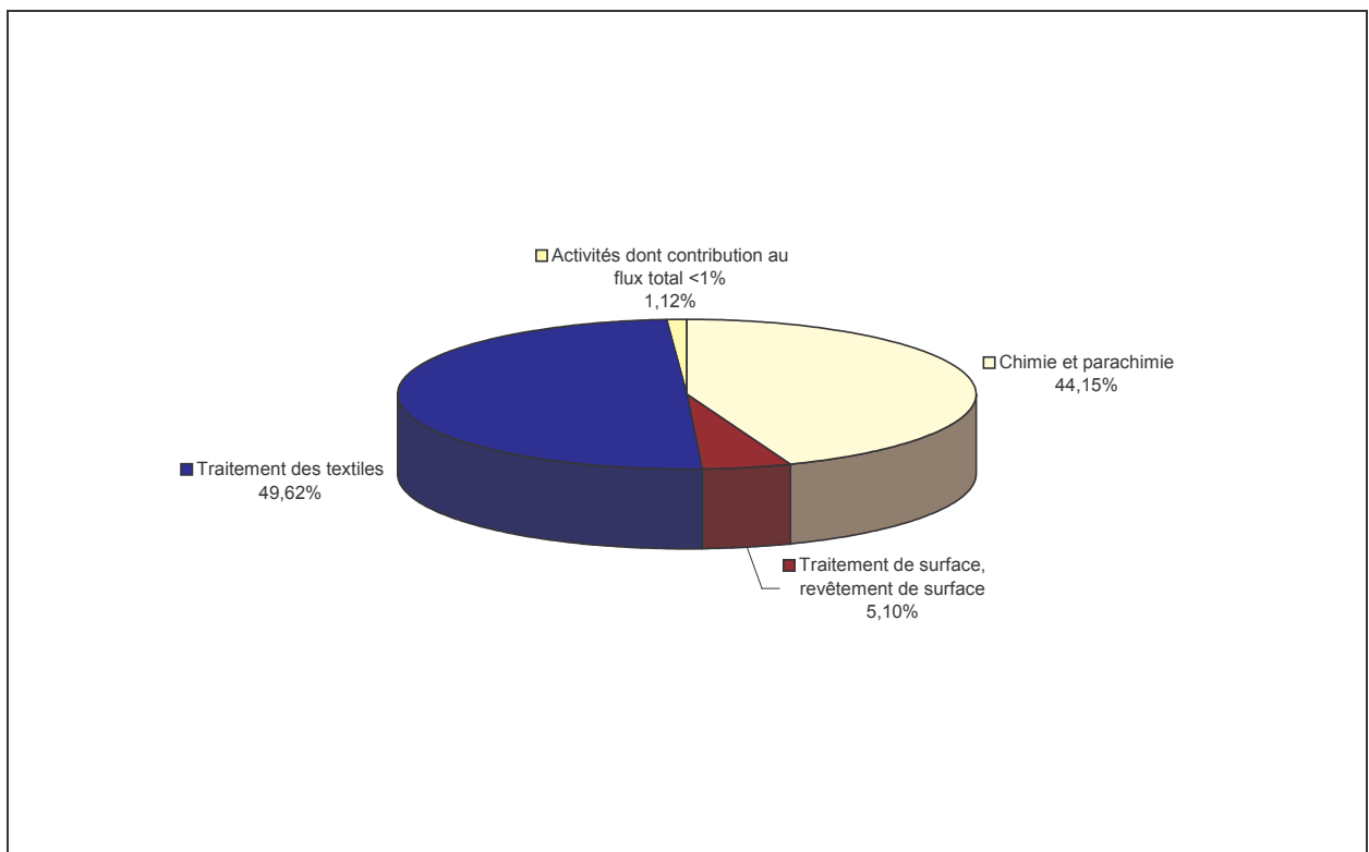
Figure 245 : Répartition par secteur d'activité des flux cumulés de d'octabromodiphenylether mesurés en sortie des sites industriels
