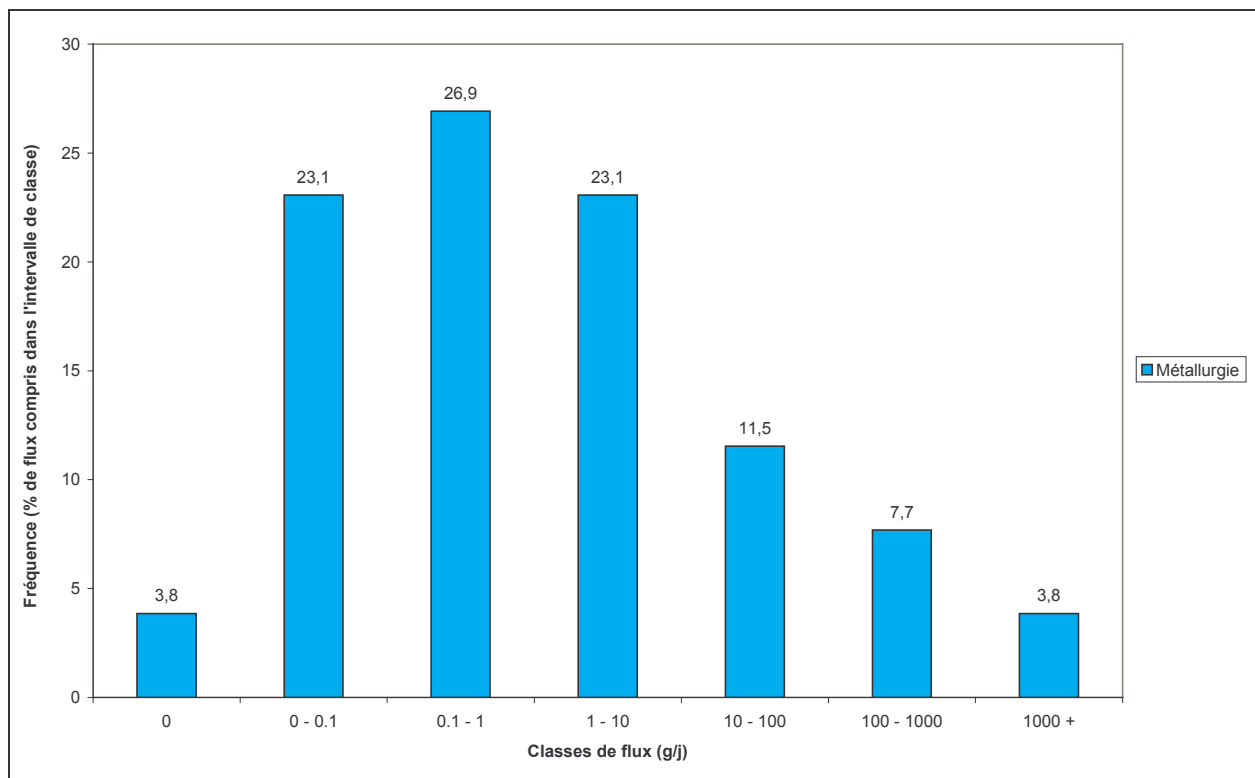
Figure 36 : Distribution des rejets industriels en fonction des flux de cadmium mesurés (secteurs d'activité contribuant à plus de 10% des émissions industrielles totales de cette substance)
