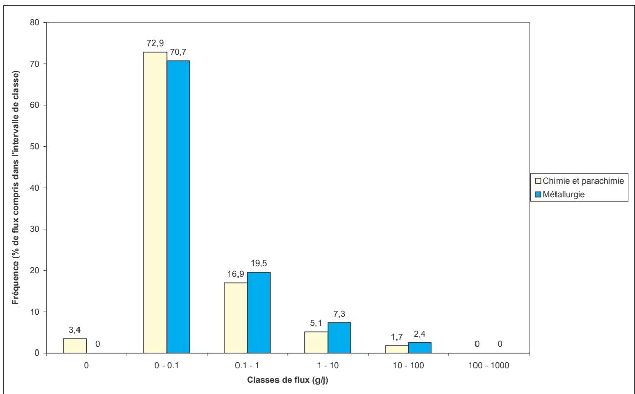
Figure 74 : Distribution des rejets industriels en fonction des flux de benzo (b) fluoranthène mesurés (secteurs d'activité contribuant à plus de 10% des émissions industrielles totales de cette substance)
