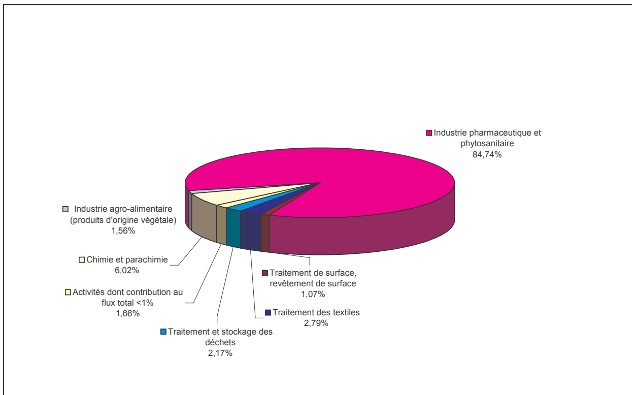
Figure 227 : Répartition par secteur d'activité des flux cumulés de 2,4 dichlorophénol mesurés en sortie des sites industriels
