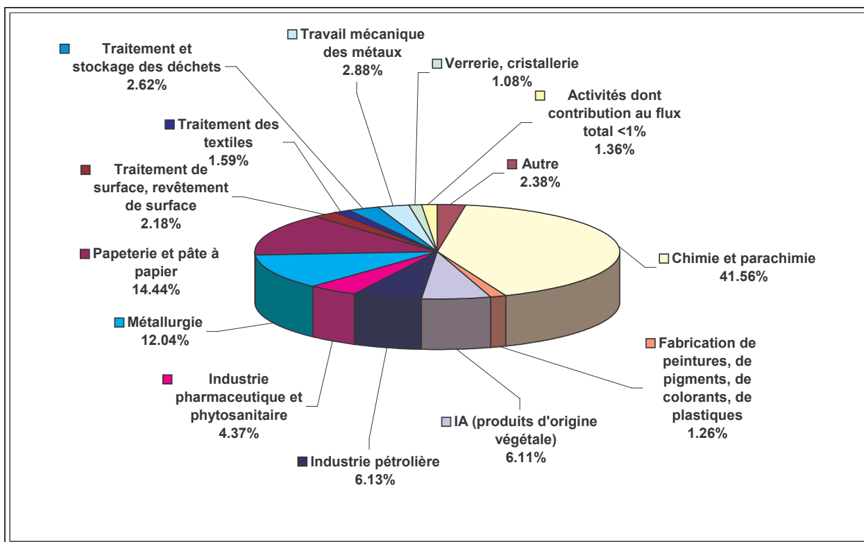
Figure 47 : Répartition par secteur d'activité des flux cumulés d'arsenic mesurés en sortie des sites industriels
