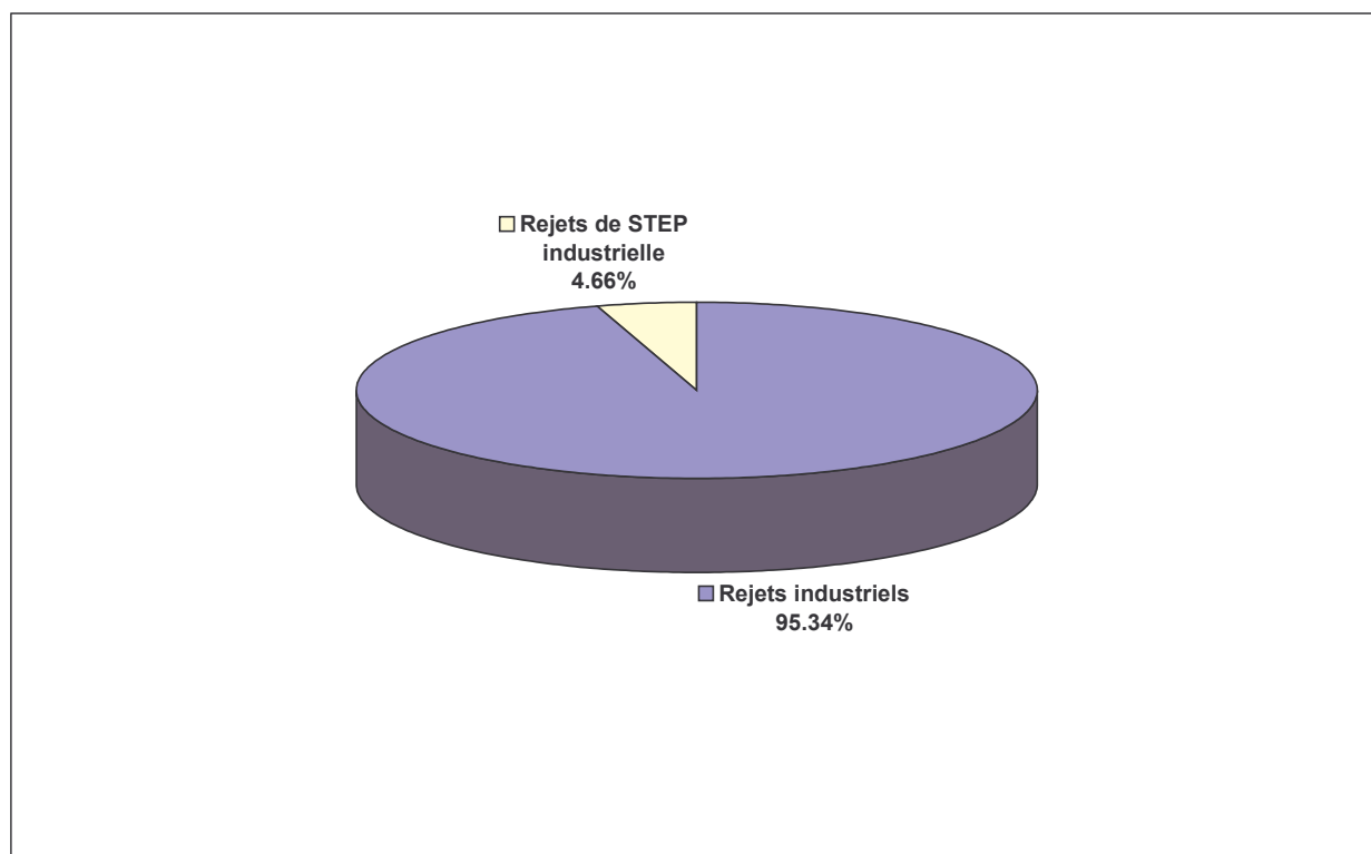
Figure 184 : Répartition des flux industriels et urbains de 1,3,5 trichlorobenzène
