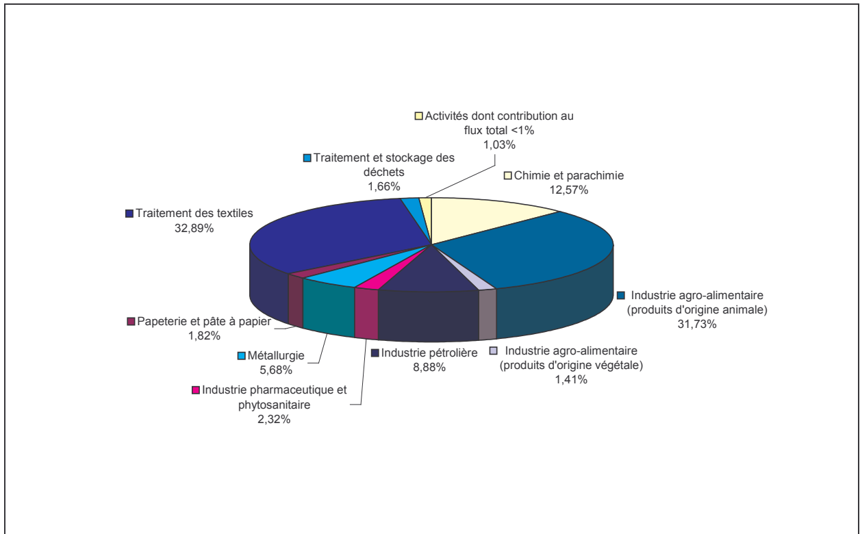
Figure 259 : Répartition par secteur d'activité des flux cumulés de chlorpyrifos mesurés en sortie des sites industriels
