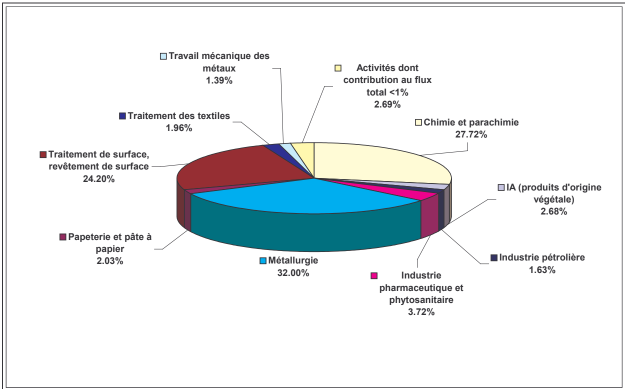
Figure 44 : Répartition par secteur d'activité des flux cumulés de nickel mesurés en sortie des sites industriels
