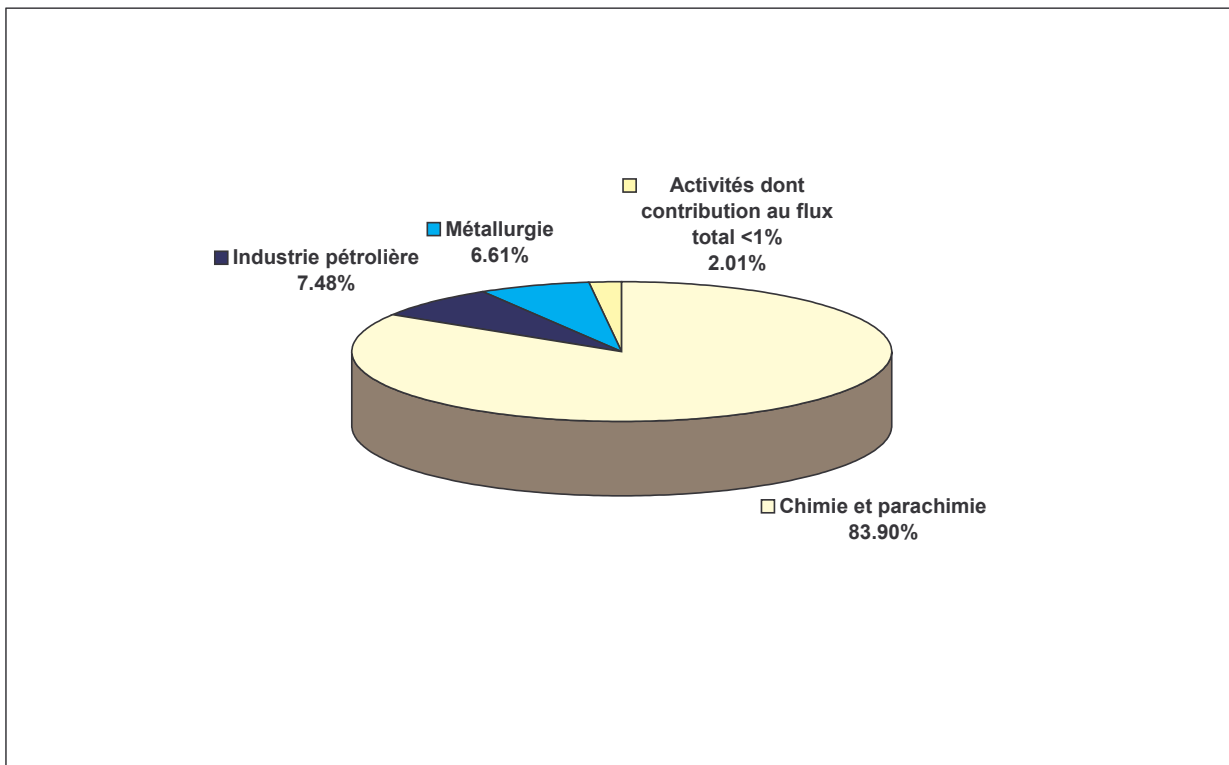
Figure 154 : Répartition par secteur d'activité des flux cumulés de benzène mesurés en sortie des sites industriels
