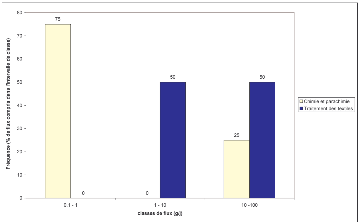
Figure 308 : Distribution des rejets industriels en fonction des flux de 4-chloro-2-nitroaniline mesurés (secteurs d'activité contribuant à plus de 10% des émissions industrielles totales de cette substance)
