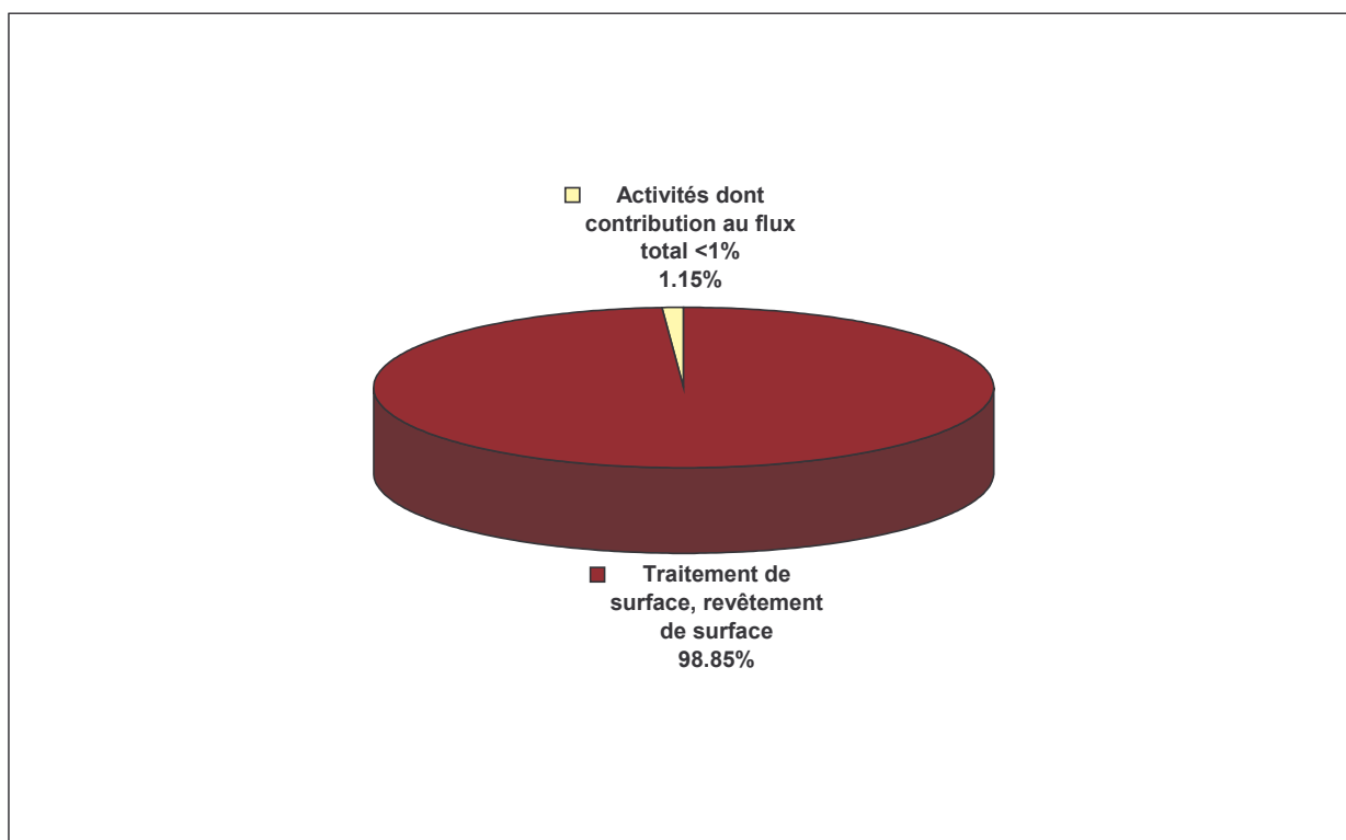
Figure 150 : Répartition par secteur d'activité des flux cumulés de chloroprène (chlorure d'allyle) mesurés en sortie des sites industriels
