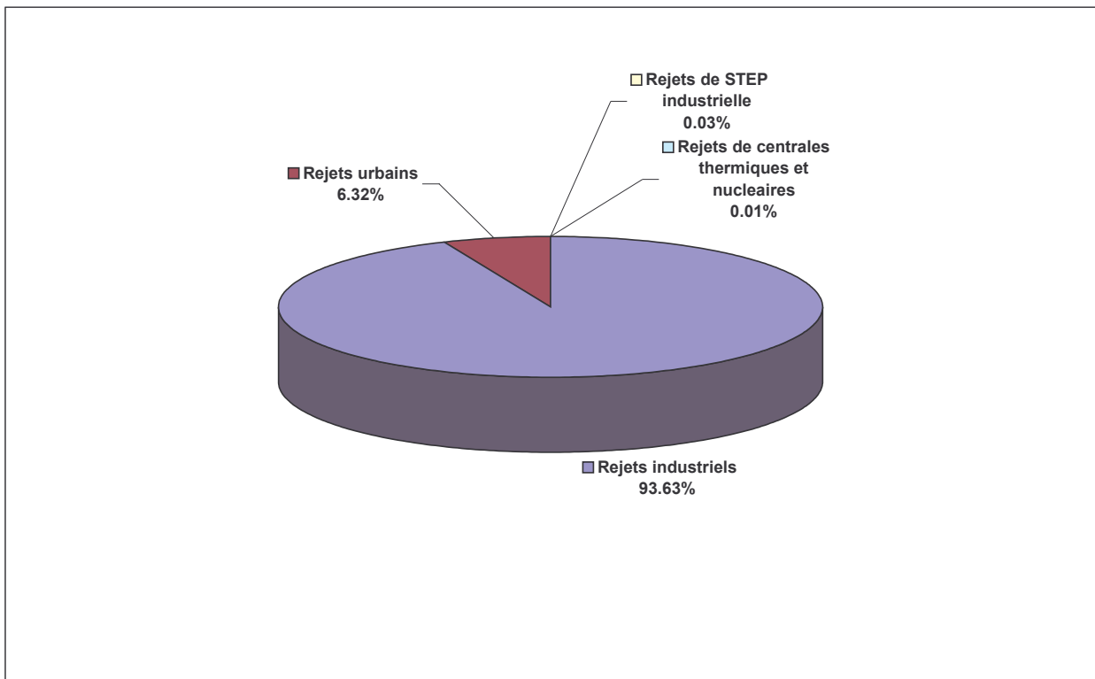
Figure 93 : Répartition des flux industriels, urbains et des CPE d'acénaphène
