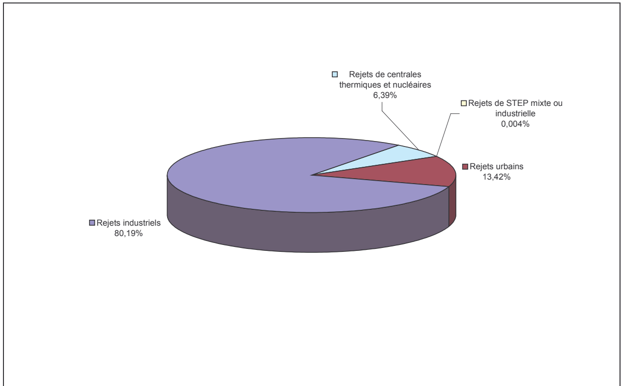
Figure 244 : Répartition des flux industriels, urbains et des CPE de d'octabromodiphenylether
