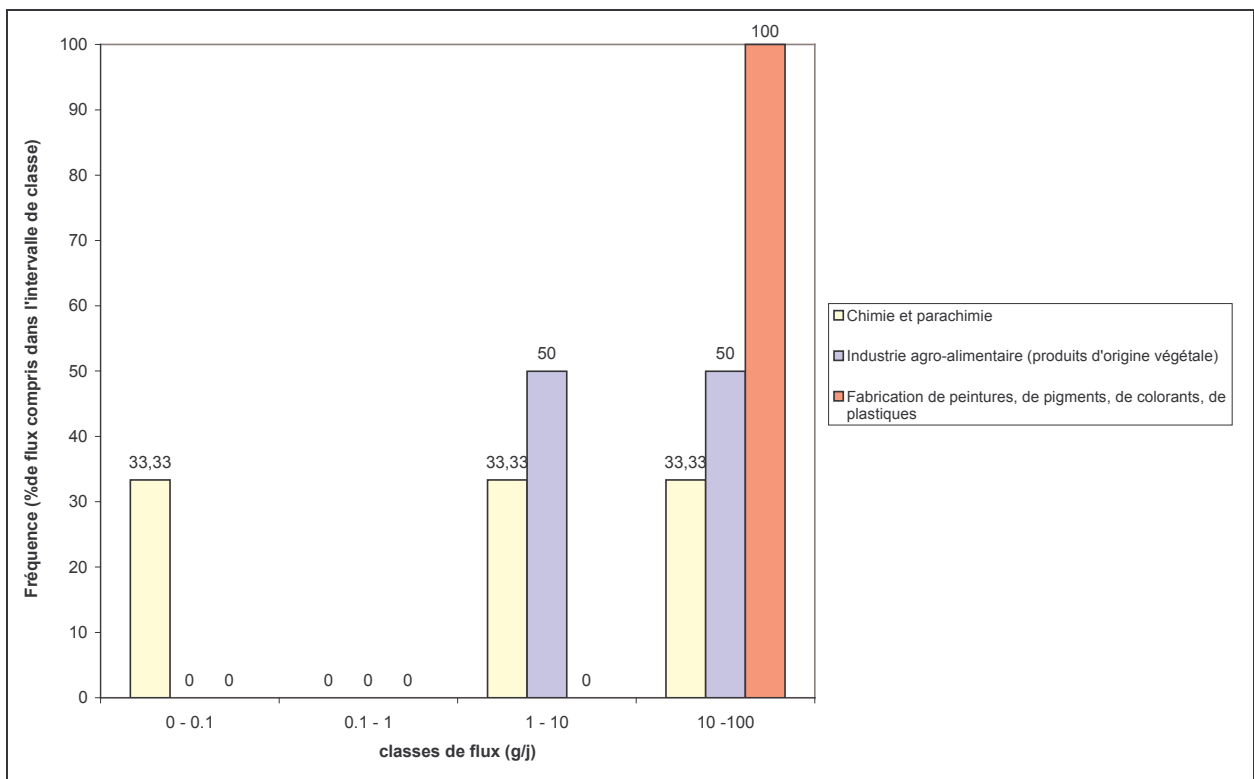
Figure 299 : Distribution des rejets industriels en fonction des flux de 3 chloroaniline mesurés (secteurs d'activité contribuant à plus de 10% des émissions industrielles totales de cette substance)
