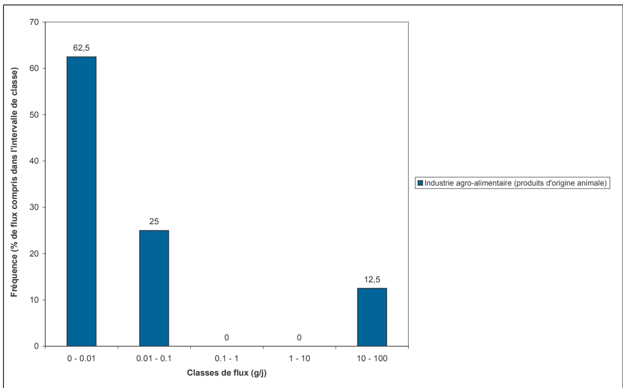
Figure 243 : Distribution des rejets industriels en fonction des flux de pentabromodiphenylether mesurés (secteurs d'activité contribuant à plus de 10% des émissions industrielles totales de cette substance)
