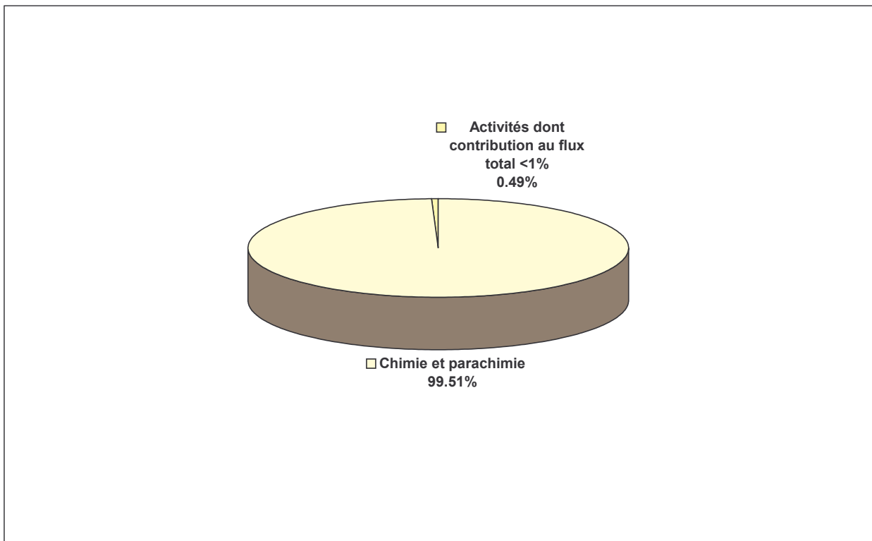
Figure 188 : Répartition par secteur d'activité des flux cumulés de pentachlorobenzène mesurés en sortie des sites industriels
