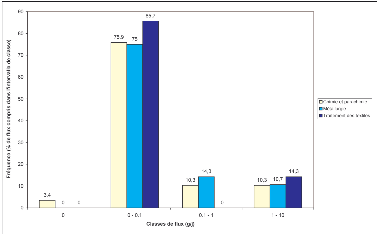
Figure 80 : Distribution des rejets industriels en fonction des flux de benzo (k) fluoranthène mesurés (secteurs d'activité contribuant à plus de 10% des émissions industrielles totales de cette substance)
