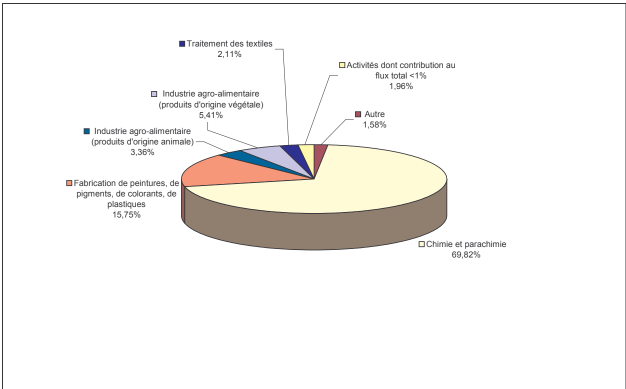
Figure 295 : Répartition par secteur d'activité des flux cumulés de 2 chloroaniline mesurés en sortie des sites industriels
