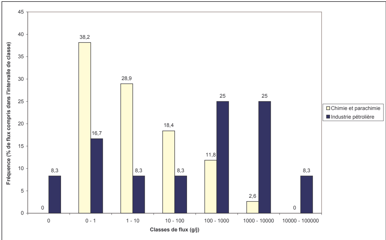
Figure 166 : Distribution des rejets industriels en fonction des flux de xylènes (somme o,p,m) mesurés (secteurs d'activité contribuant à plus de 10% des émissions industrielles totales de cette substance)
