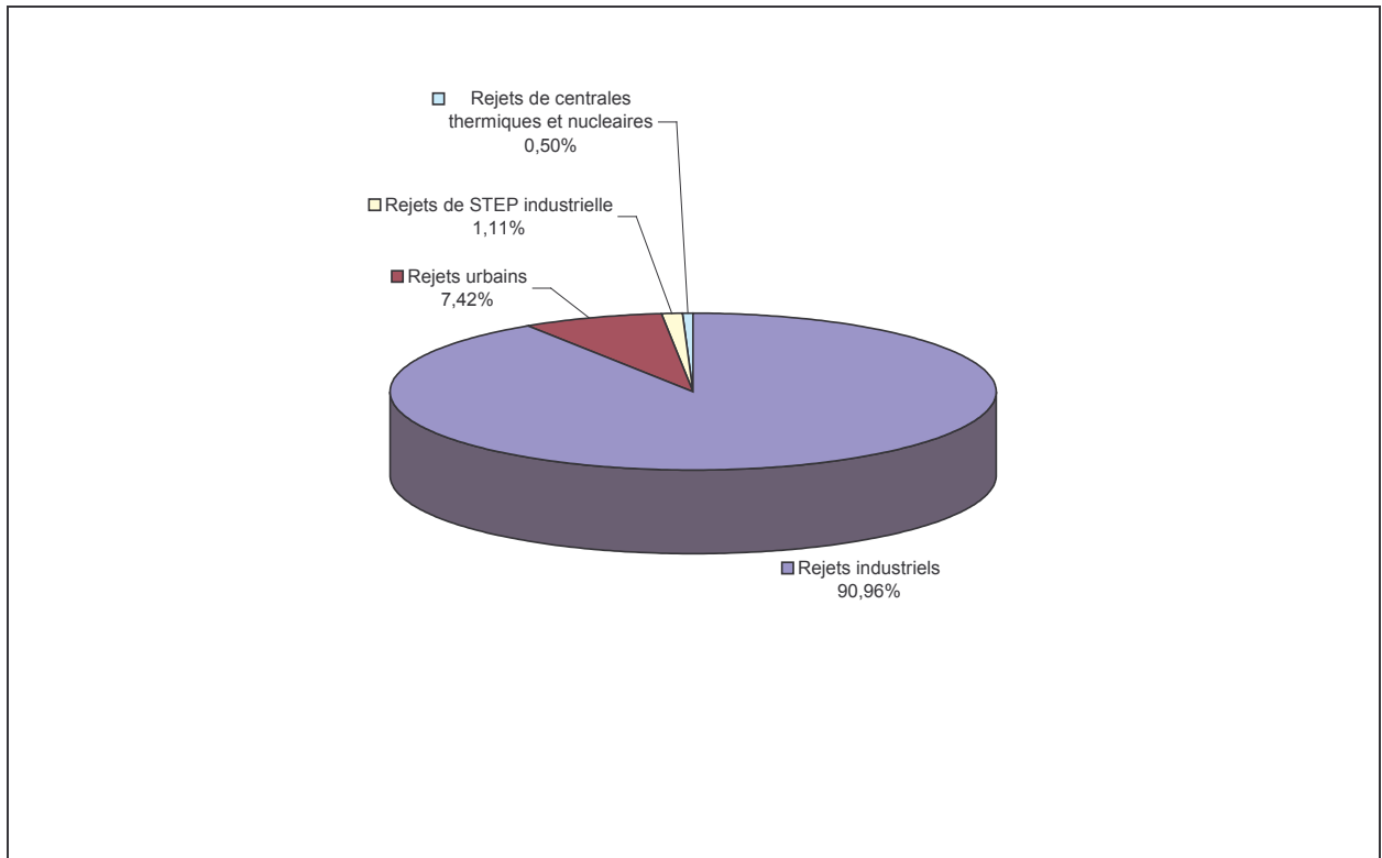
Figure 213 : Répartition des flux industriels, urbains et des CPE de para-tert-octylphénol
