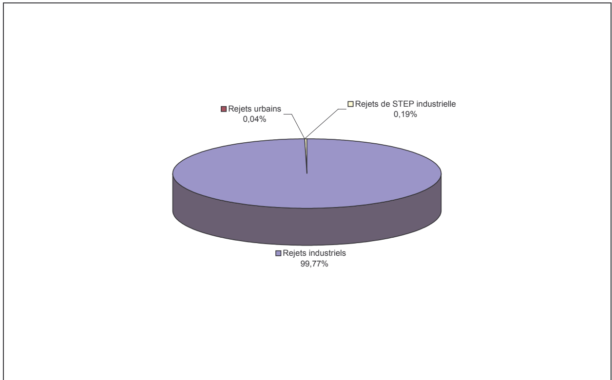
Figure 291 : Répartition des flux industriels et urbains de biphényle
