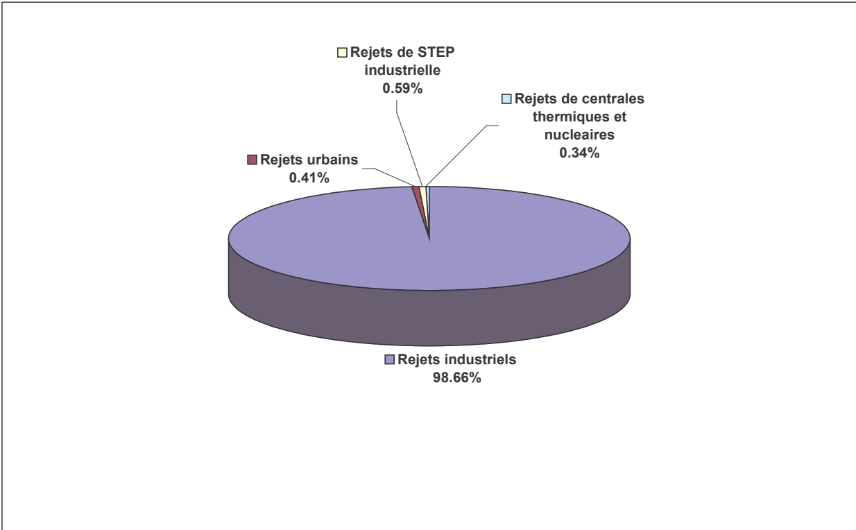
Figure 87 : Répartition des flux industriels, urbains et des CPE de naphtalène
