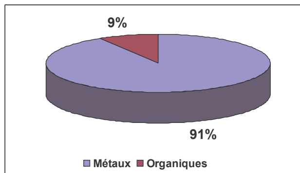
Figure 342 : Répartition des flux de substances organiques et métalliques mesurés en sortie des sites secteur d'activité TS
