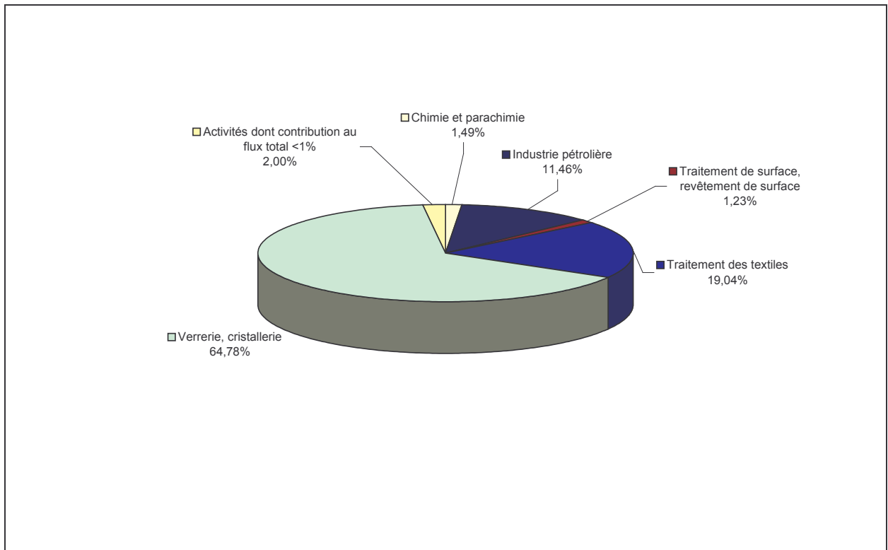
Figure 292 : Répartition par secteur d'activité des flux cumulés de biphényle mesurés en sortie des sites industriels
