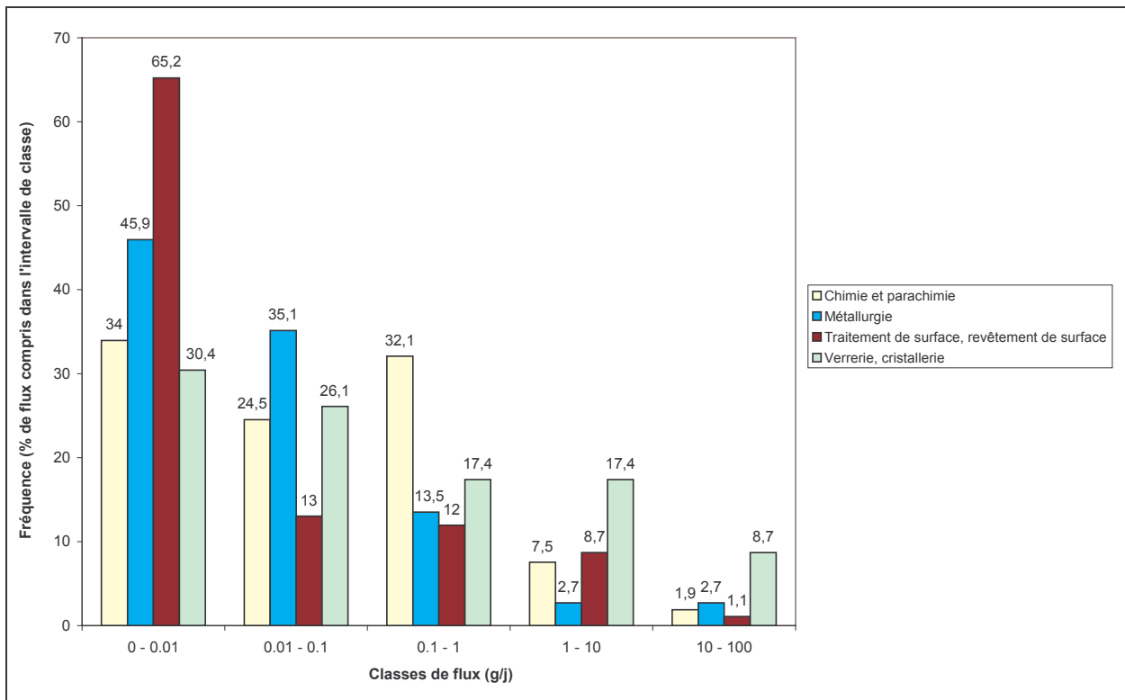
Figure 63 : Distribution des rejets industriels en fonction des flux de monobutylétain cation mesurés (secteurs d'activité contribuant à plus de 10% des émissions industrielles totales de cette substance)
