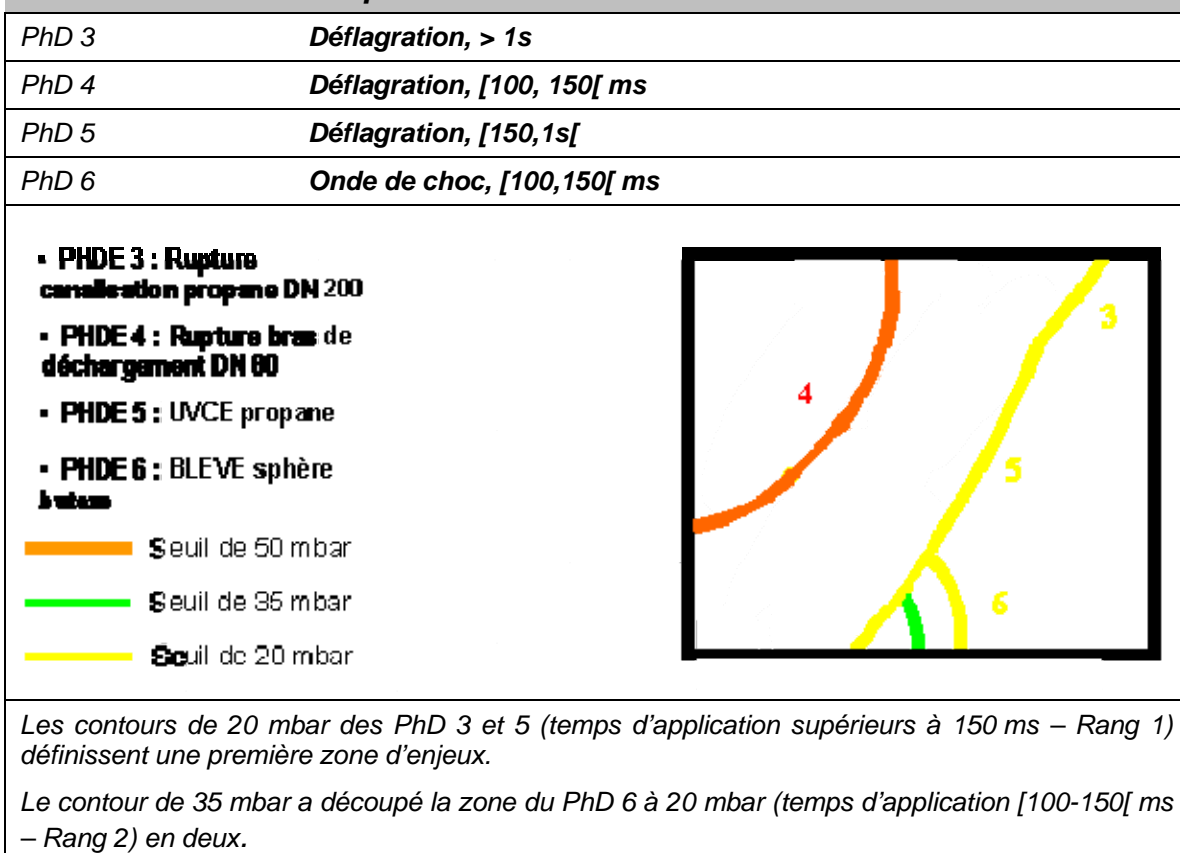
Figure 4 : Exemple de découpage par le contour 35 mbar sur les zones d'enjeux en 20-50 mbar
