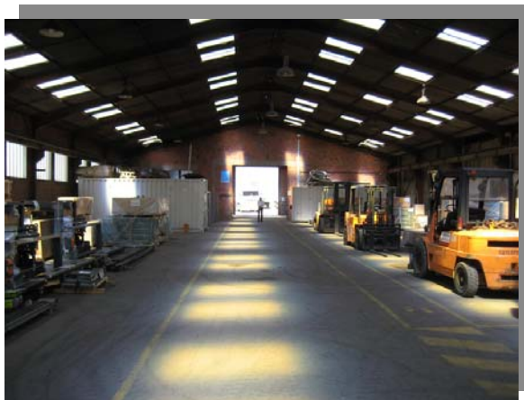
Figure 35 : Entrepôts dont la portée des poutres fermières est supérieure à 13 m (Source : INERIS)
